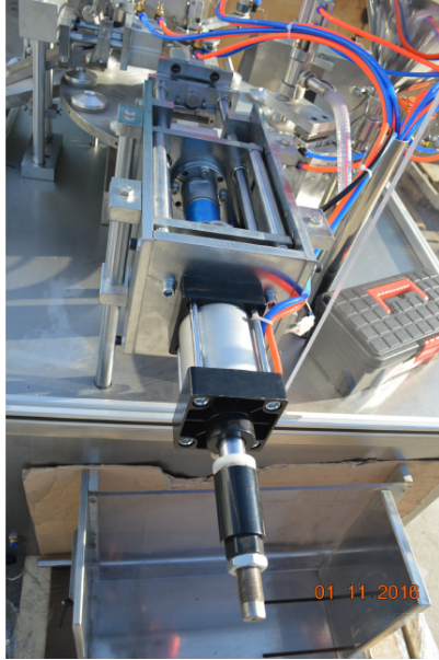
Tolva: Sistema de Llenado de la Bomba de Pistón:
